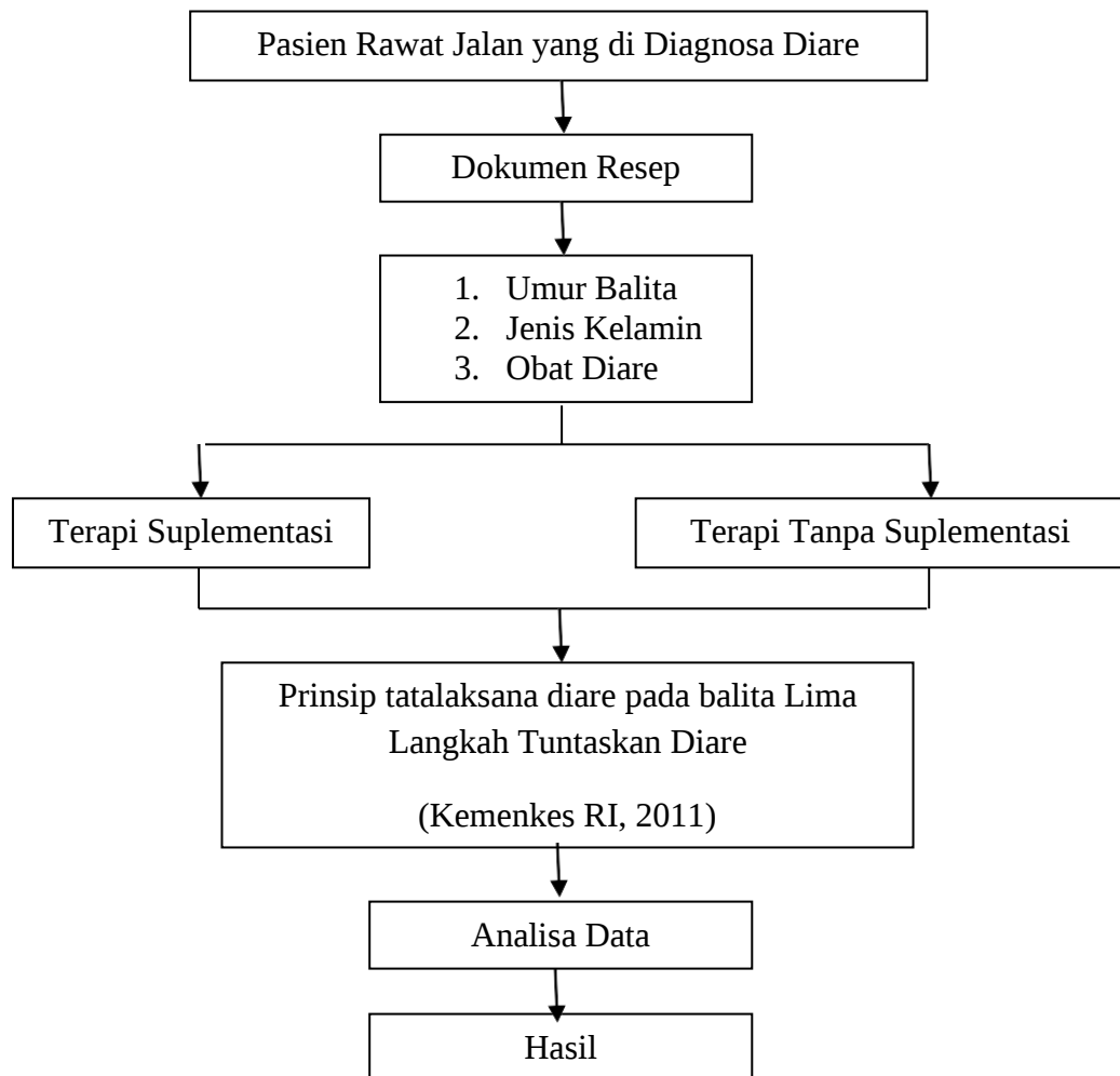
Gambar III.1 Kerangka Konsep
