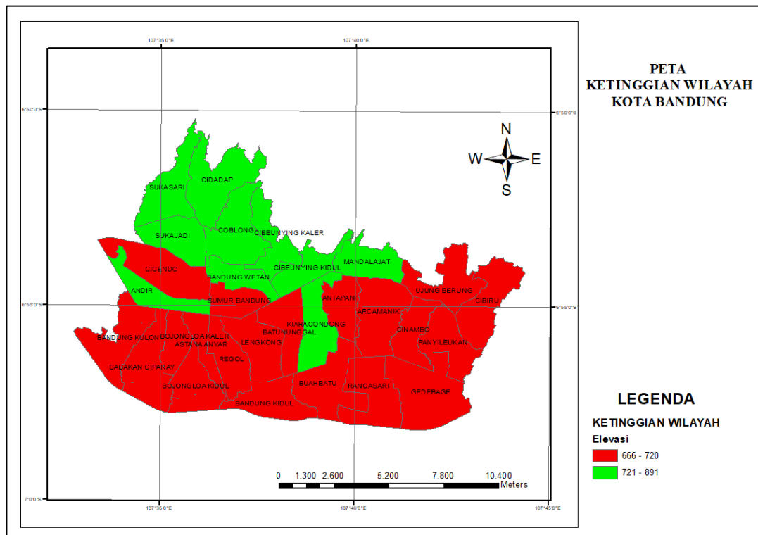
Lampiran 27. Peta Sebaran Ketinggian Wilayah Kota Bandung Tahun 2019-2023
