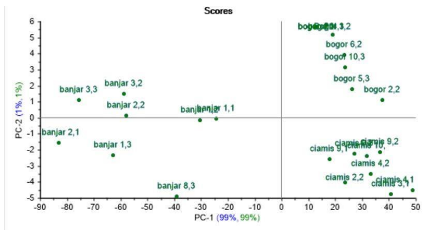
Lampiran VIII. Hasil dari Plot PCA cross validation
