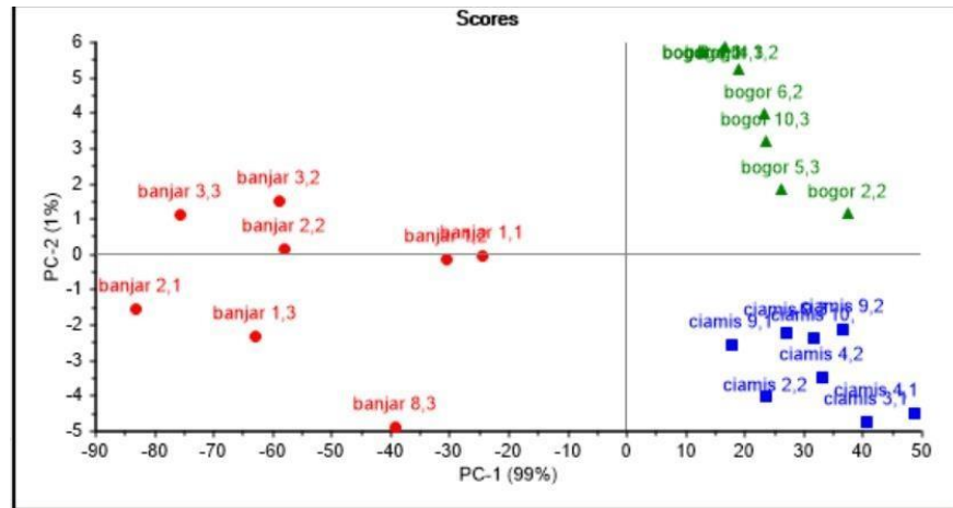
Lampiran VII. Hasil Score plot PCA menggunakan kombinasi baseline dan smoothing .
