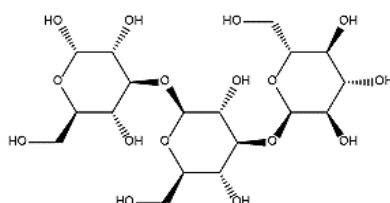
Laminarin
