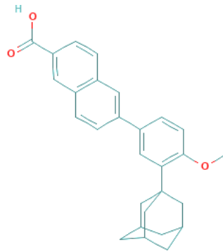
Gambar II.9 : Struktur kimia Adapalene
