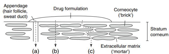
Gambar II.3 : Jalur permeasi obat di kulit (stratum korneum)
