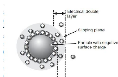
Gambar II.8 : Electric double layer mengelilingi nanopartikel (Eptember & Iego, 2012).
